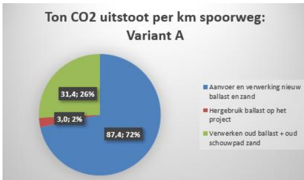
Figuur 6: Cirkeldiagram CO 2 -uitstoot variant A enkel (4Infra, 2025)
